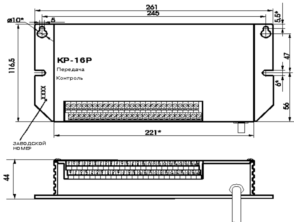
Рис.1 Габаритно-присоединительные размеры КР-16Р
