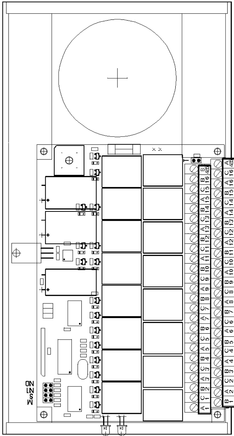
Рис.2 Плата контроллера при снятой верхней крышке с указанием назначения клемм и перемычек.
