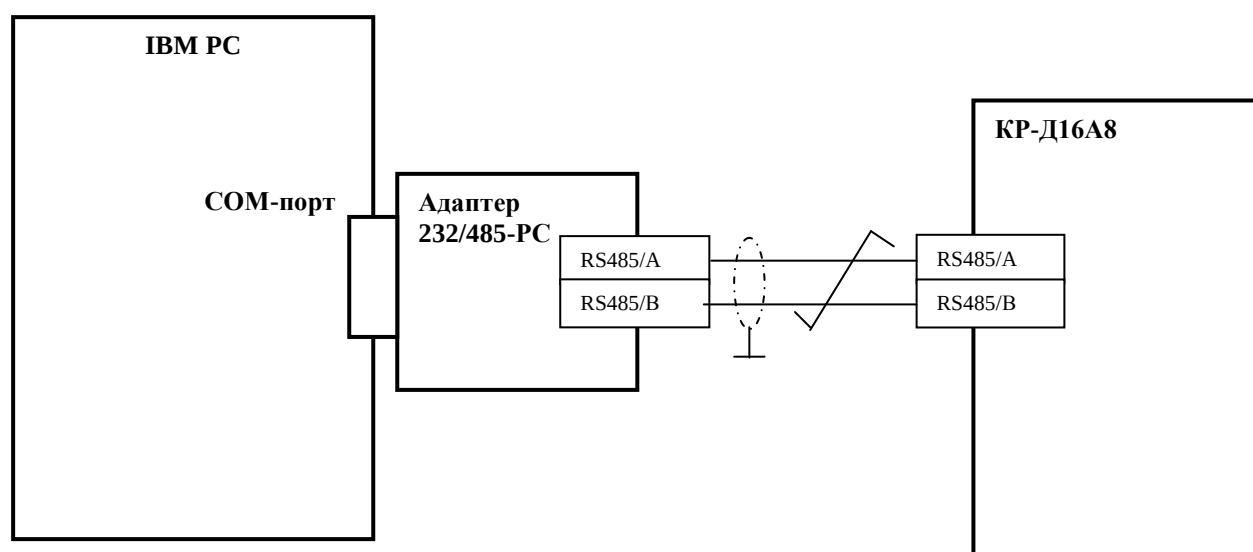
Рис.5 Подключение КР к компьютеру при изменении настроек
