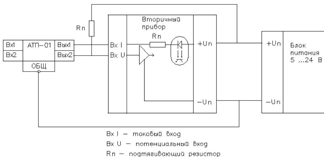
Рис.5. Подключение адаптера к другим вторичным приборам
